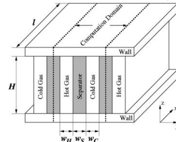
Figure 1. A schematic model of the micro heat exchanger. mHEX 内部における支配方程式は下記の通りである。
